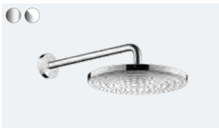
Raindance Select S hoofddouche 300 2jet met douche-arm # 27378, -000, -400 17 l/min hoofddouche 300 2jet met plafondaansluiting (zonder afb.) # 27337, -000, -400 17 l/min
